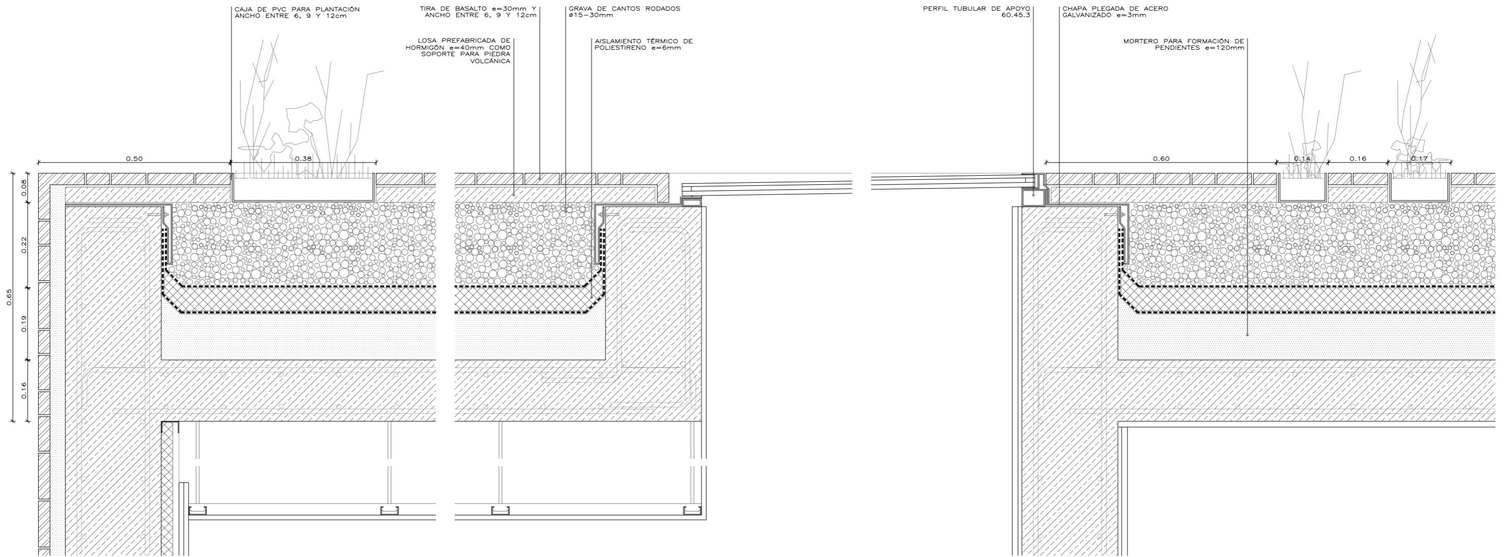
SECCIÓN LONGITUDINAL DE CUBIERTA \frac{0}{0,2M}
