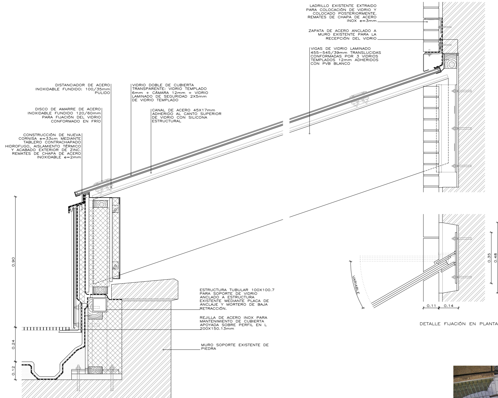
DETALLE APOYO EN CUBIERTA 0 0,3M
