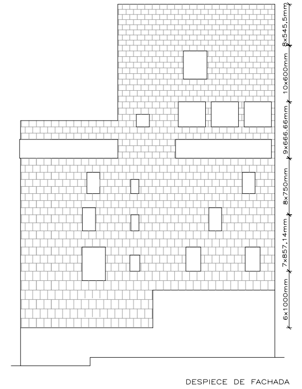
DESPIECE DE FACHADA
