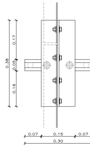
ALZADO DE ANCLAJE 0 0,2M
