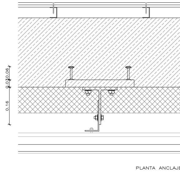
PLANTA ANCLAJE
