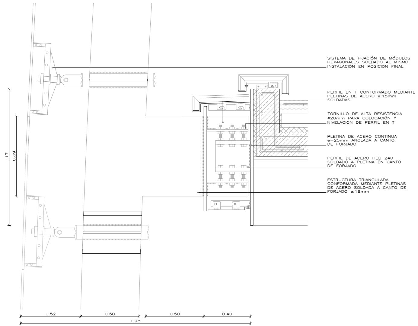
DETALLE SECCIÓN 0 0,4M
