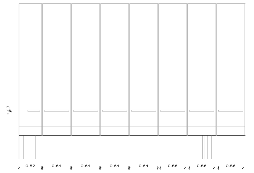
DETALLE ALZADO
