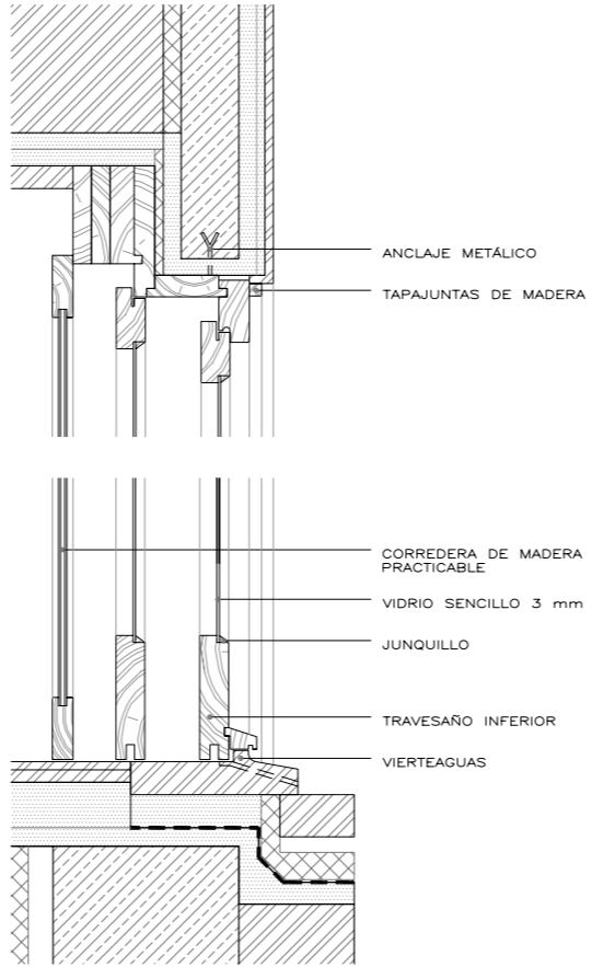
DETALLE SECCIÓN
