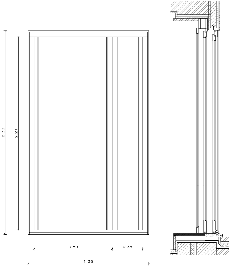
ALZADO
