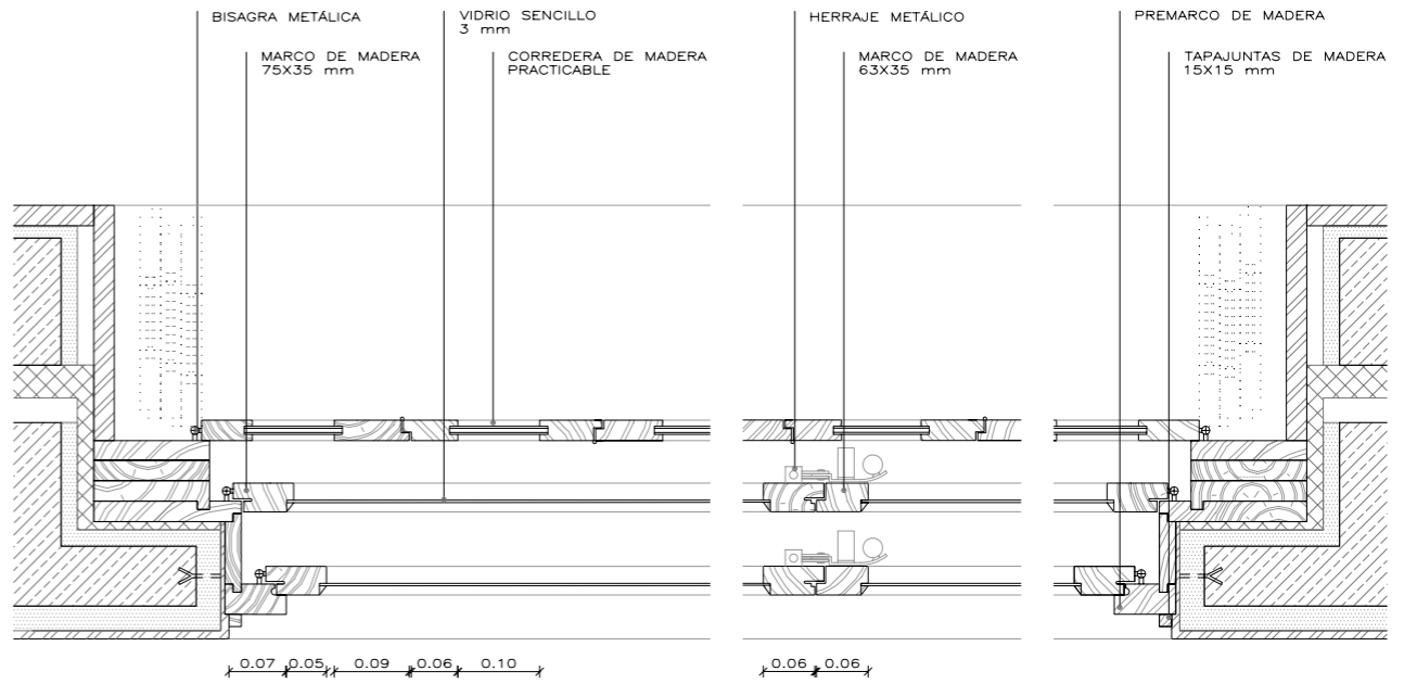
DETALLE PLANTA 0 0,2M
