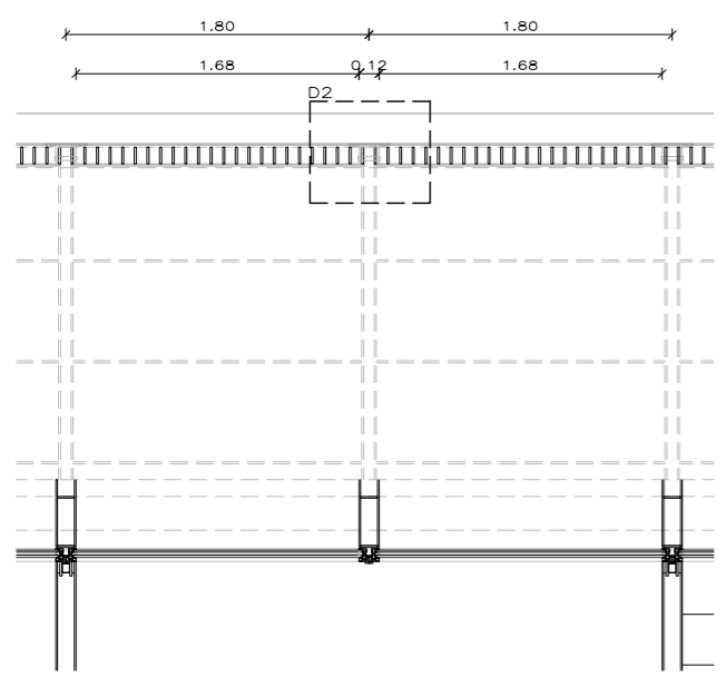
PLANTA 0 1 M
