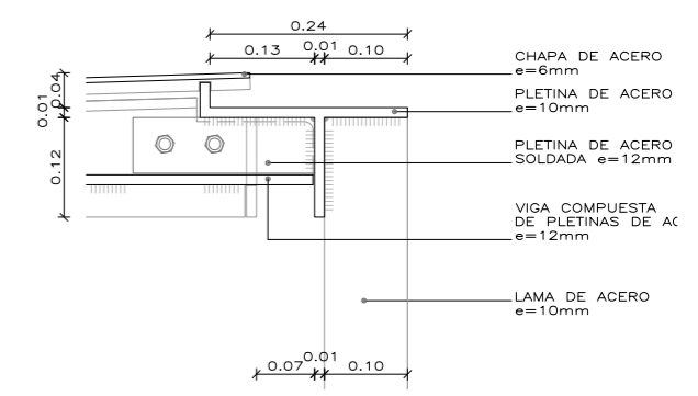
SECCIÓN D-1.2
