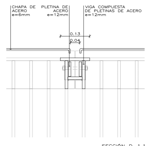
SECCIÓN D-1.1
