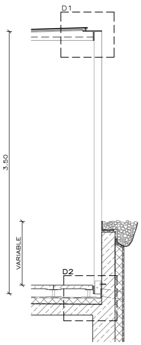
SECCIÓN
