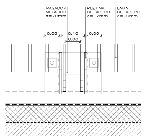
SECCIÓN D-2.1
