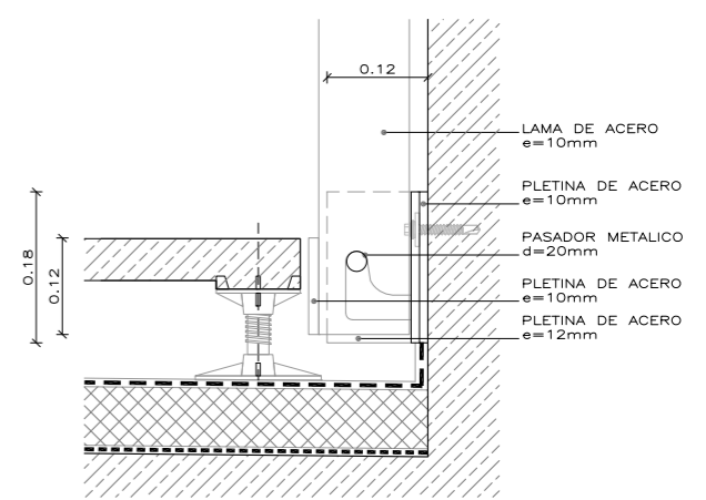
SECCIÓN D-2.2 0 0.2 M
