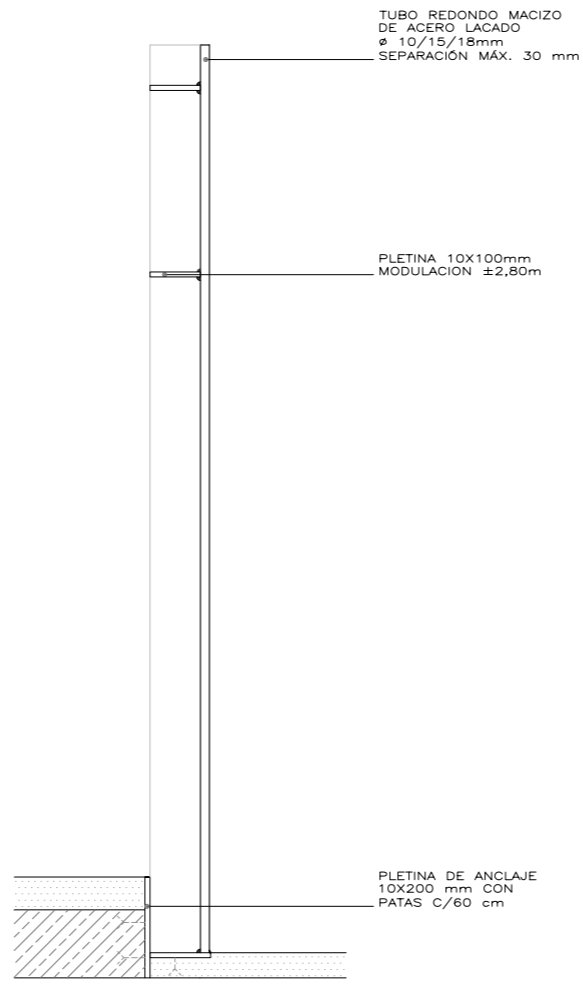
SECCIÓN
