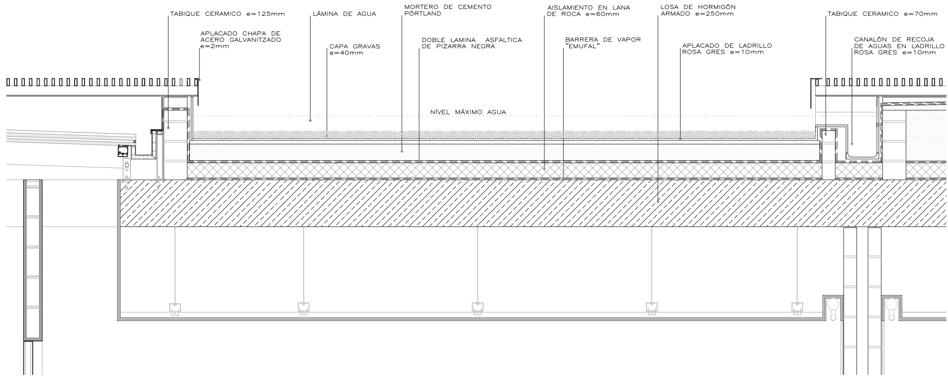
D1-DETALLE SECCIÓN TRANSVERSAL 0 0,4M
