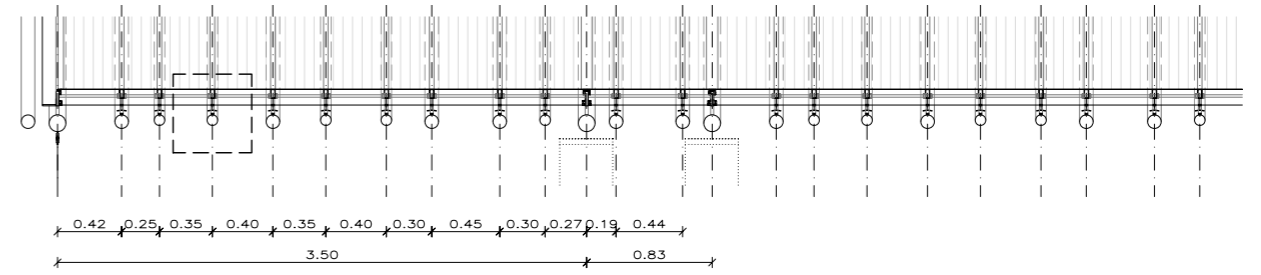
SECCION TRANSVERSAL 0 1M
