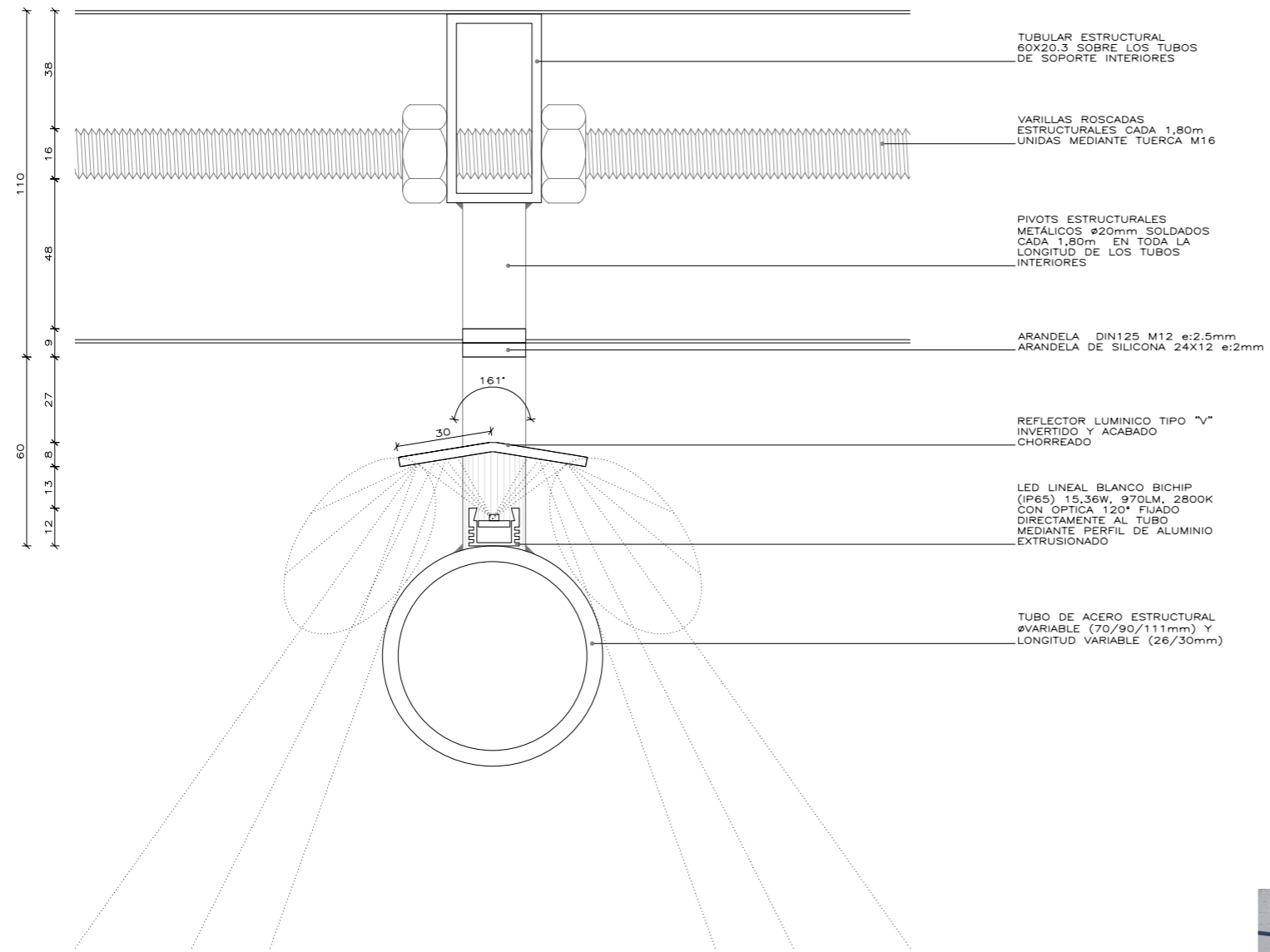
DETALLE COLOCACIÓN LED LINEAL 0 0,05M
