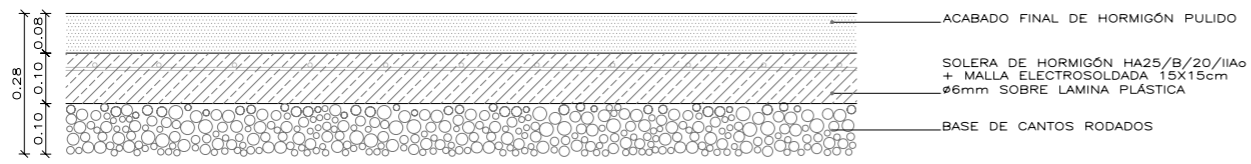
PAVIMENTO DE COCINA 0 0,3M
