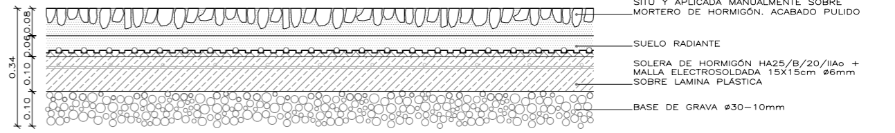
PAVIMENTO DE COMEDOR 0 0,3M
