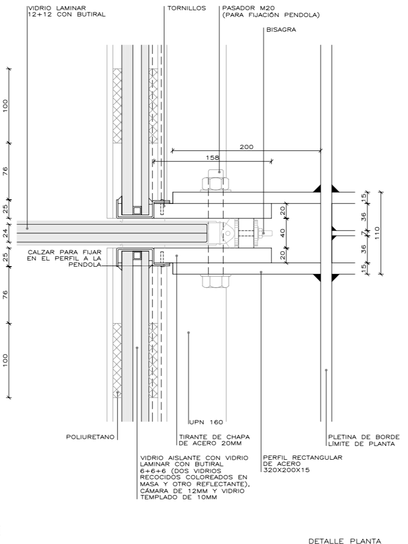
DETALLE PLANTA
