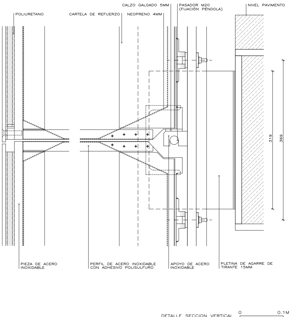
DETALLE SECCION VERTICAL 0 0.1M
