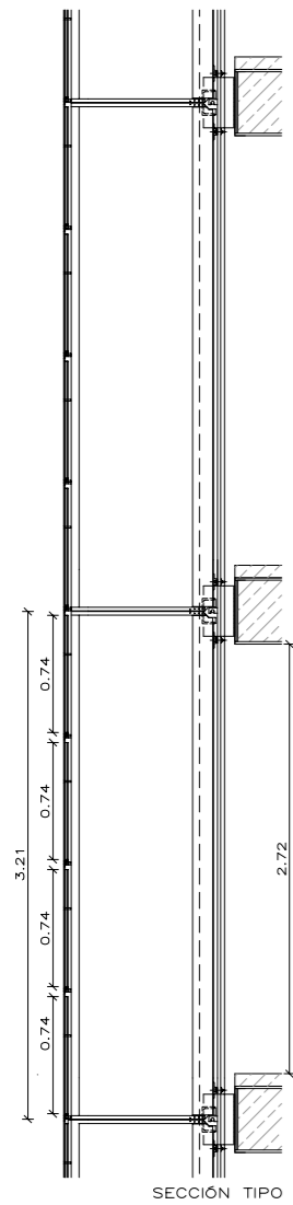
SECCIÓN TIPO
