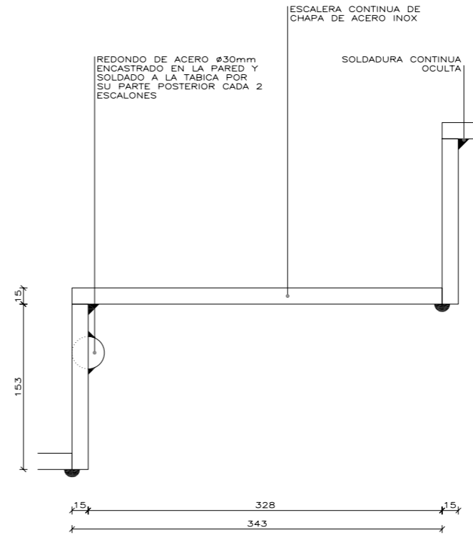
DETALLE ESCALÓN LONGITUDINAL
