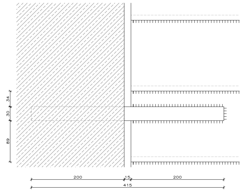
DETALLE ANCLAJE A LA PARED 0 0.04M
