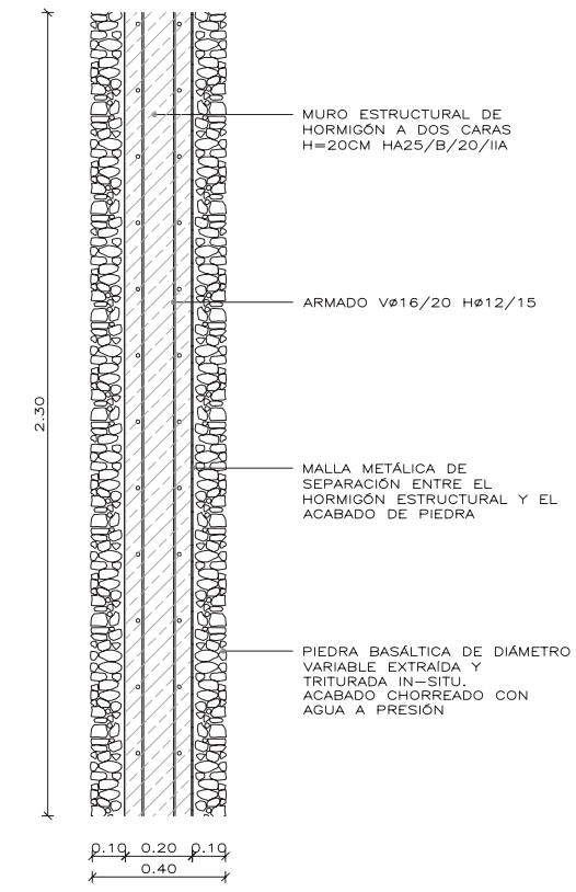
DETALLE SECCIÓN VERTICAL 0 0,5M
