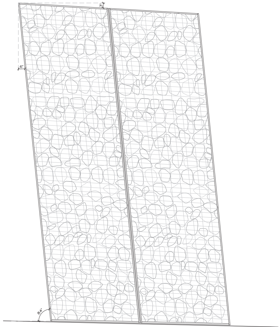
ALZADO
