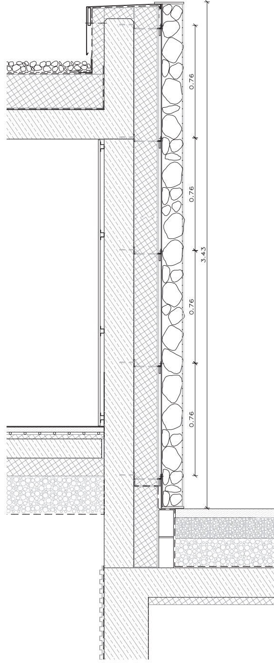
SECCIÓN
