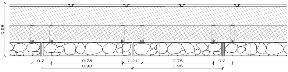
PLANTA 0 0,4M
