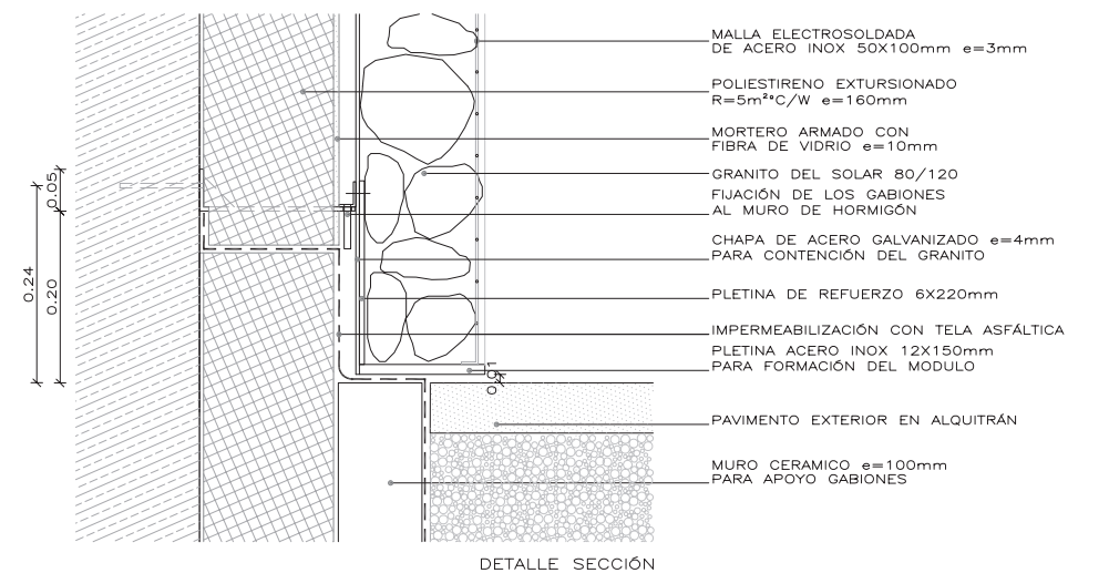
DETALLE SECCIÓN
