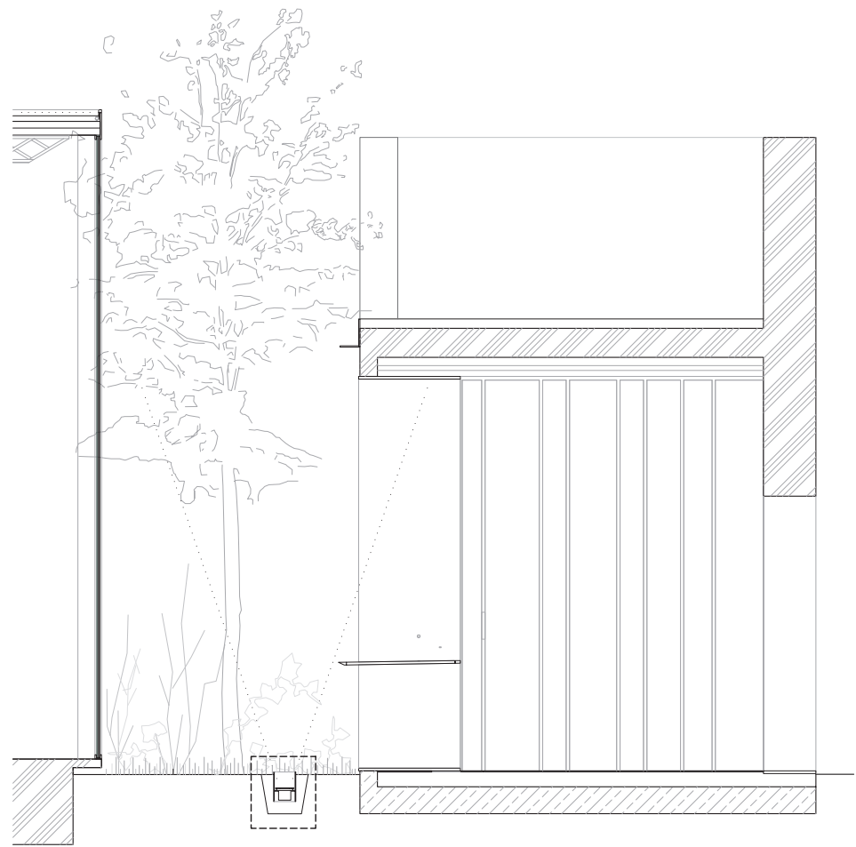
SECCIÓN UBICACIÓN LUMINÁRIA 0 1M
