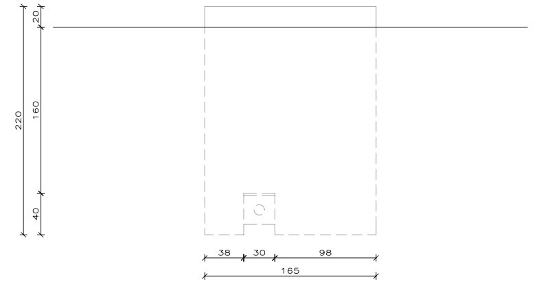
DETALLE COLOCACIÓN LUMINÁRIA ALZADO
