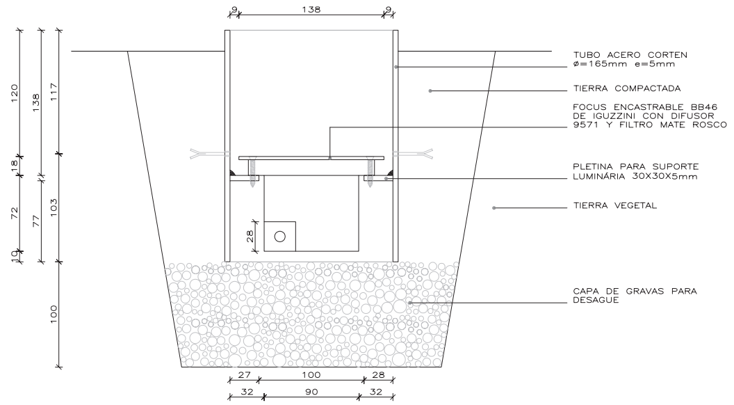
DETALLE COLOCACIÓN LUMINÁRIA SECCIÓN
